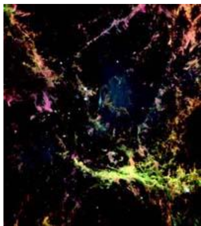
蟹状星云（照片由 NASA 提供）
