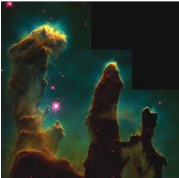
鹰状星云
