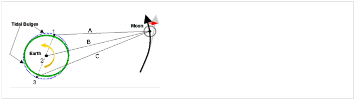
图 2. 月球目前的退行速度
